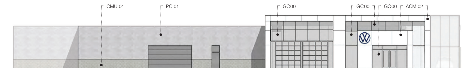
D East Elevation SCAL- : // 01 = 1461
