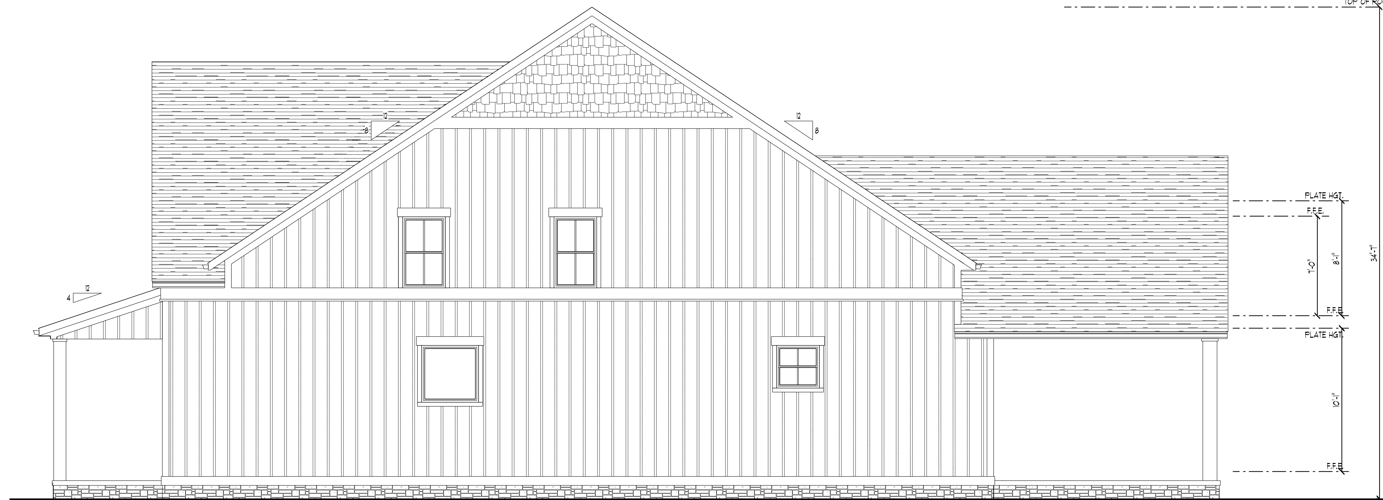
RIGHT ELEVATION
