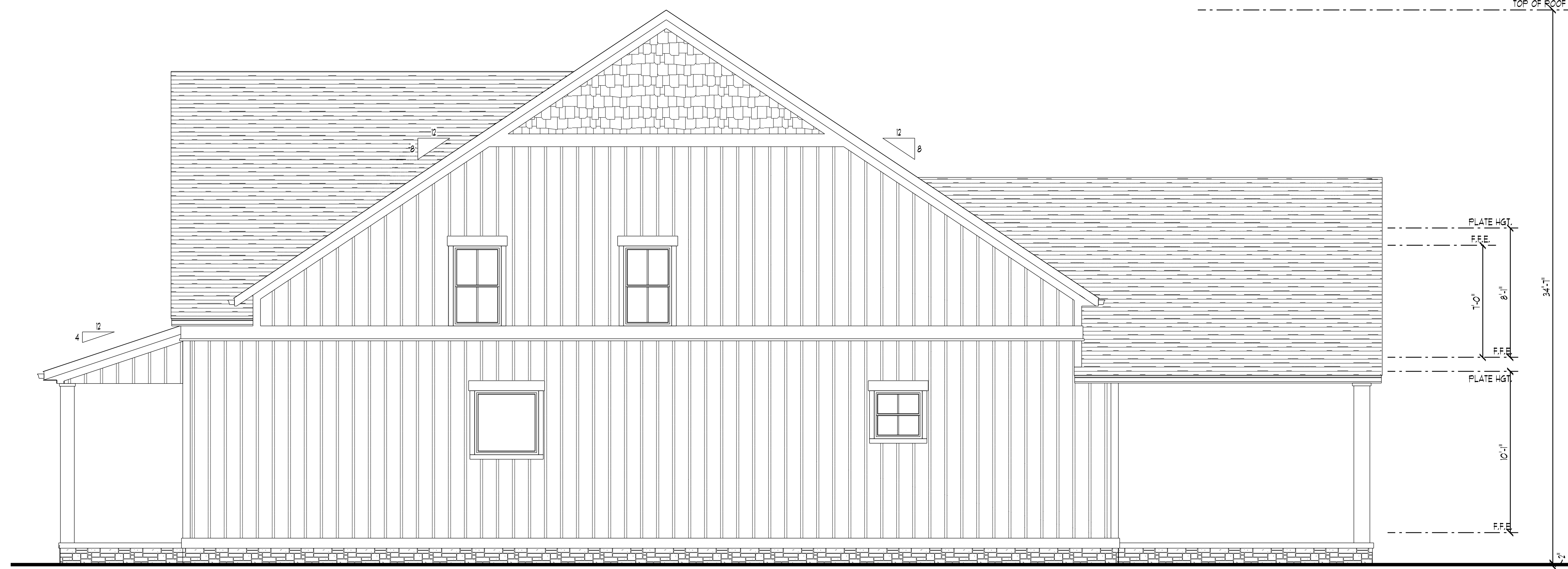
RIGHT ELEVATION
